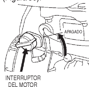
Figura 30. Interruptor ON/OFF ENCENDIDO/APAGADO (Posición OFF APAGADO)
