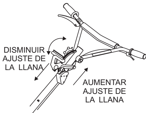
Figura 29. Mango en T con Quick-Pitch™
