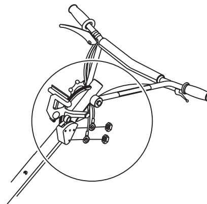
Figura 14. Conexión del cableado
