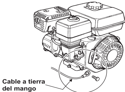
Figura 11. Conexión del cable a tierra
