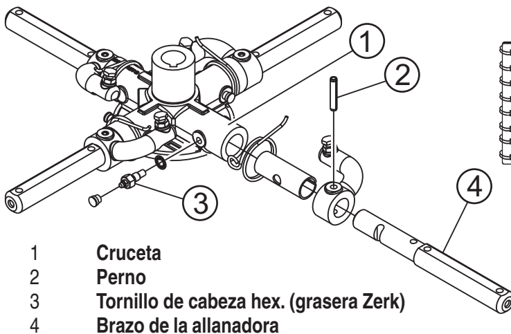
Figura 43. Retirando el perno y la grasera Zerk
