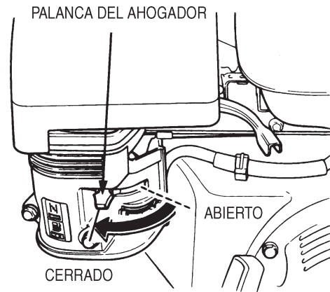
Figura 26. Palanca del ahogador del motor
