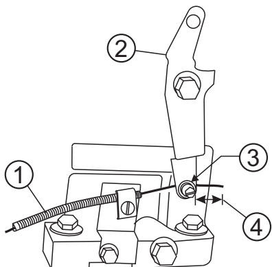
Figura 7. Conexión del cable del acelerador (HONDA)
