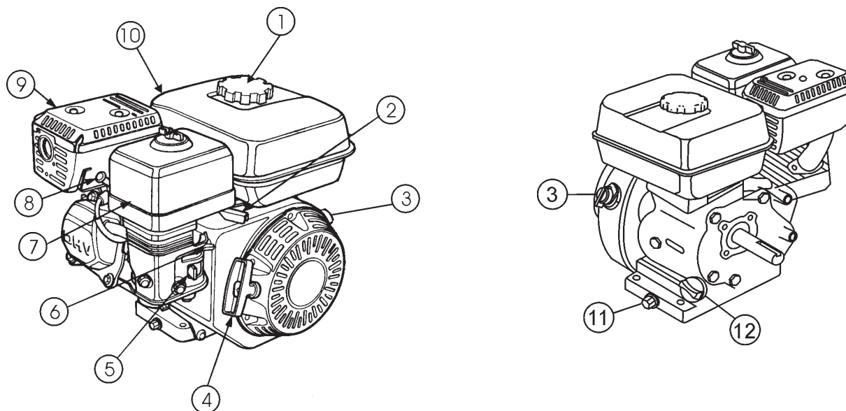
Figura 4. Controles y componentes del motor
