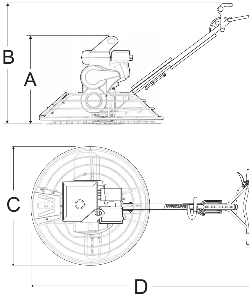
Figura 1. Dimensiones de la allanadora J-36/M-30
