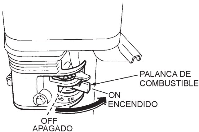
Figura 24. Palanca de la válvula de combustible del motor
