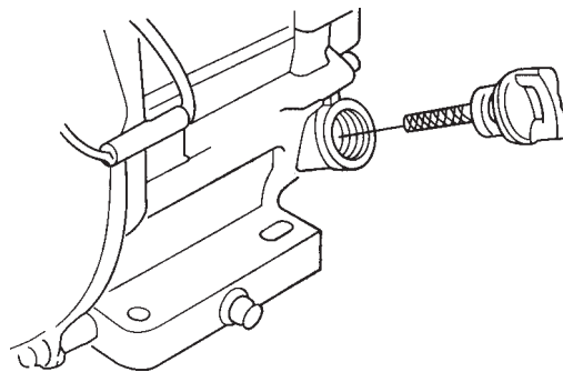
Figura 19. Varilla medidora del aceite del motor (Extracción)
