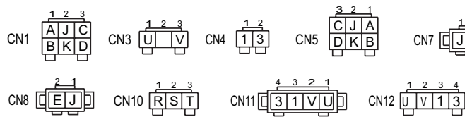
ARRANGEMENT DE CONNECTEUR (AFFICHAGE DE L'INSTALLATION)
