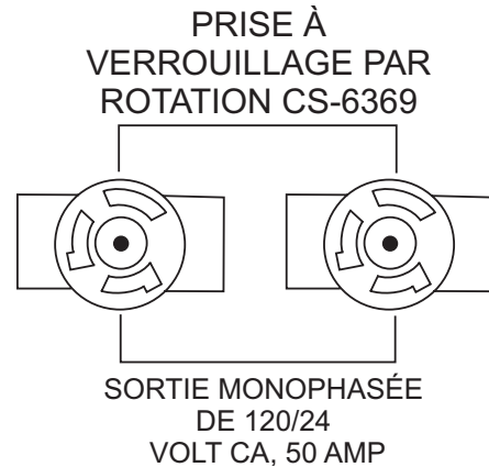
Figure 8. Prises de 120/240 VAC à Verrouillage par Rotation
