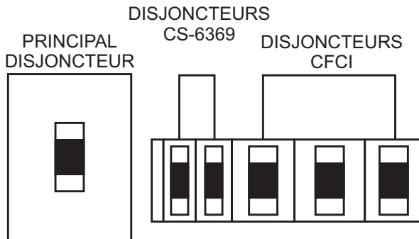
Figure 26. Disjoncteur Principal, GFCI ou Auxiliaire (OFF)
