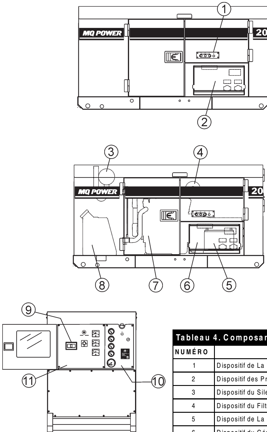
Figure 3. Composants majeurs
