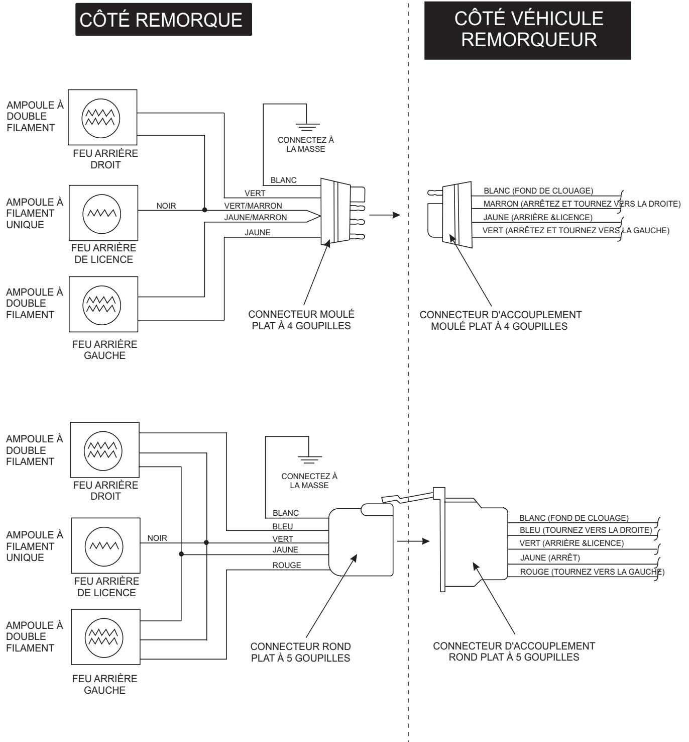
Figure 45. Schéma de Câblage du Véhicule de Remorquage/de la Remorque
