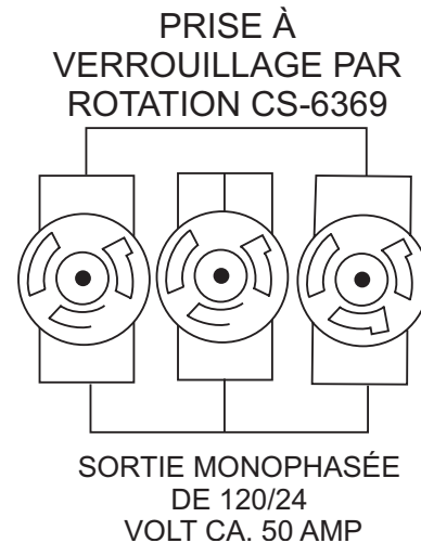
Figure 8. Prises de 120/240 VAC à Verrouillage par Rotation
