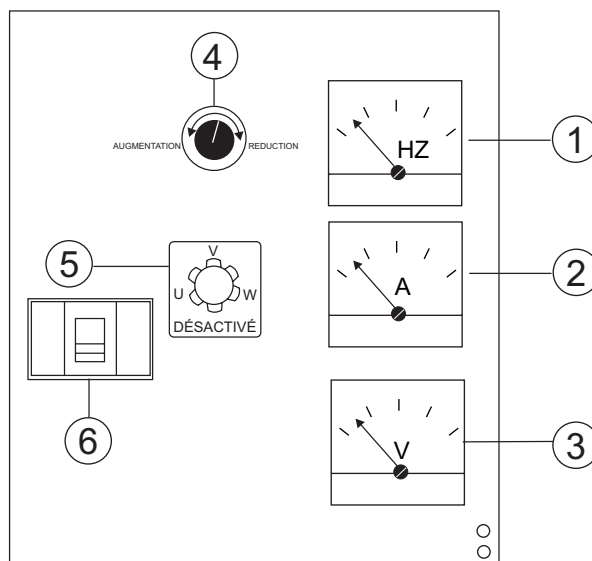
Figure 4. Panneau de Commande du Générateur
