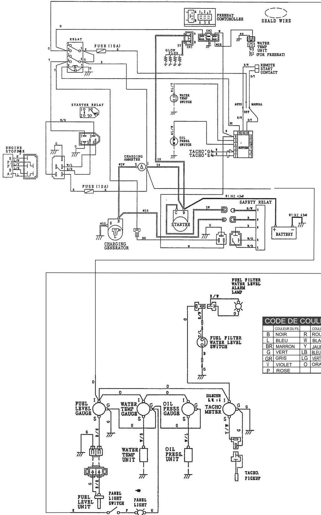
Figure 47 : Schéma de Câblage du Moteur
