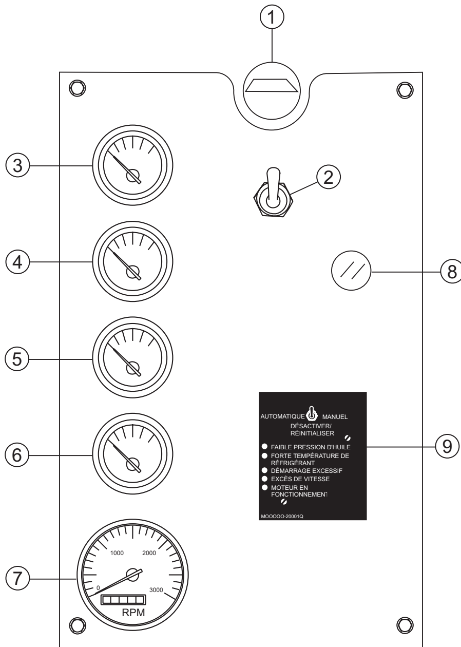
Figure 5. Panneau de Fonctionnement du Moteur
