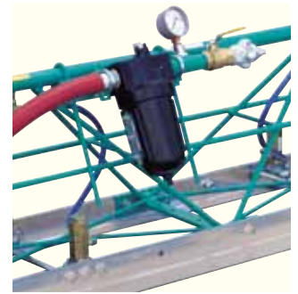
El regulador de aire y el lubricador de neblina hacen que los vibradores del pistón funcionen en condiciones óptimas. (Se incluyen con el kit de manilla de extremo WSHAH.)
