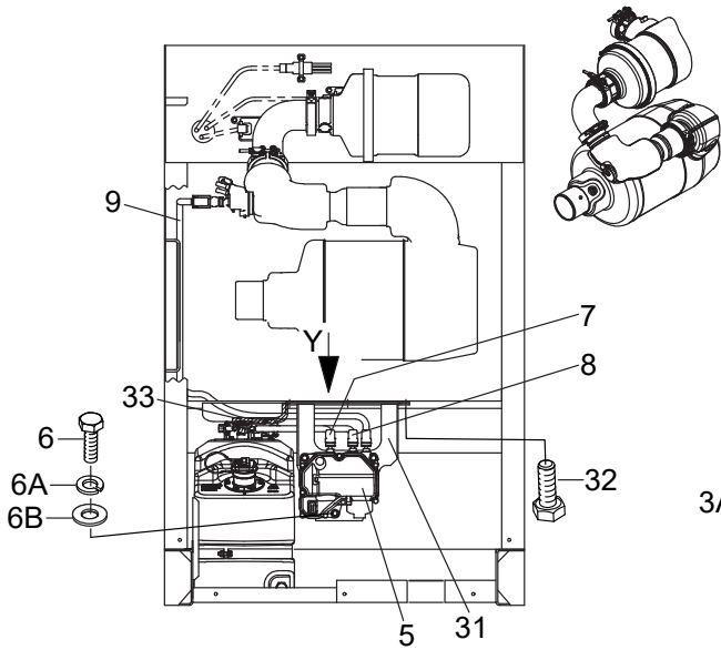
VIEW - Y
