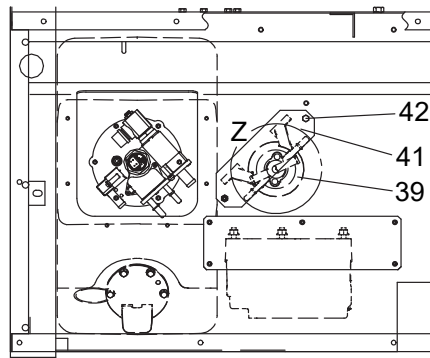
VIEW - Y
